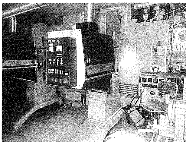
2-es fénykép: A jobboldali mozigép áttekintő fényképe (12964)
