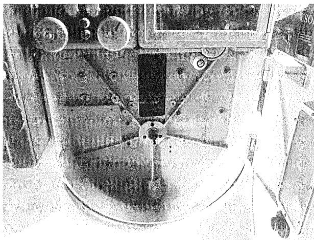
8-as fénykép: Az aldoboz és abban az olajszivárgás
