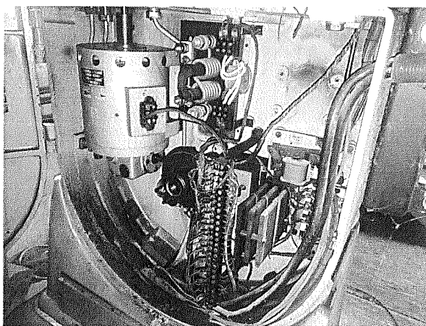
9-es fénykép: Az aldobozzal szembeni elektromos szekrény és az olajszivárgás
