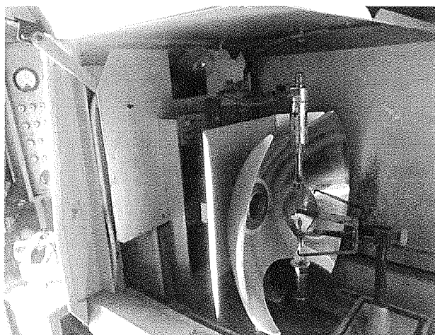
14-es fénykép: A xenon ívláma a projektorházban
